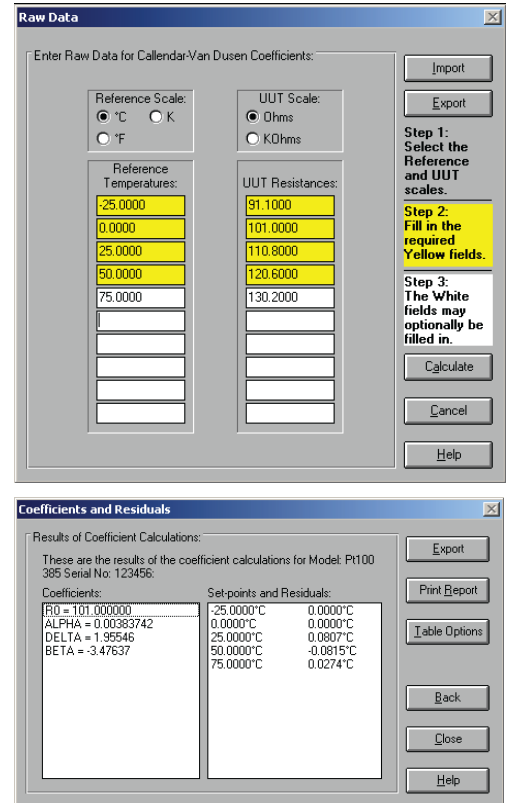
图 6. 福禄克计量校准部的 TableWare 软件计算独有的 CVD 常数，使其与探头特征相一致。
